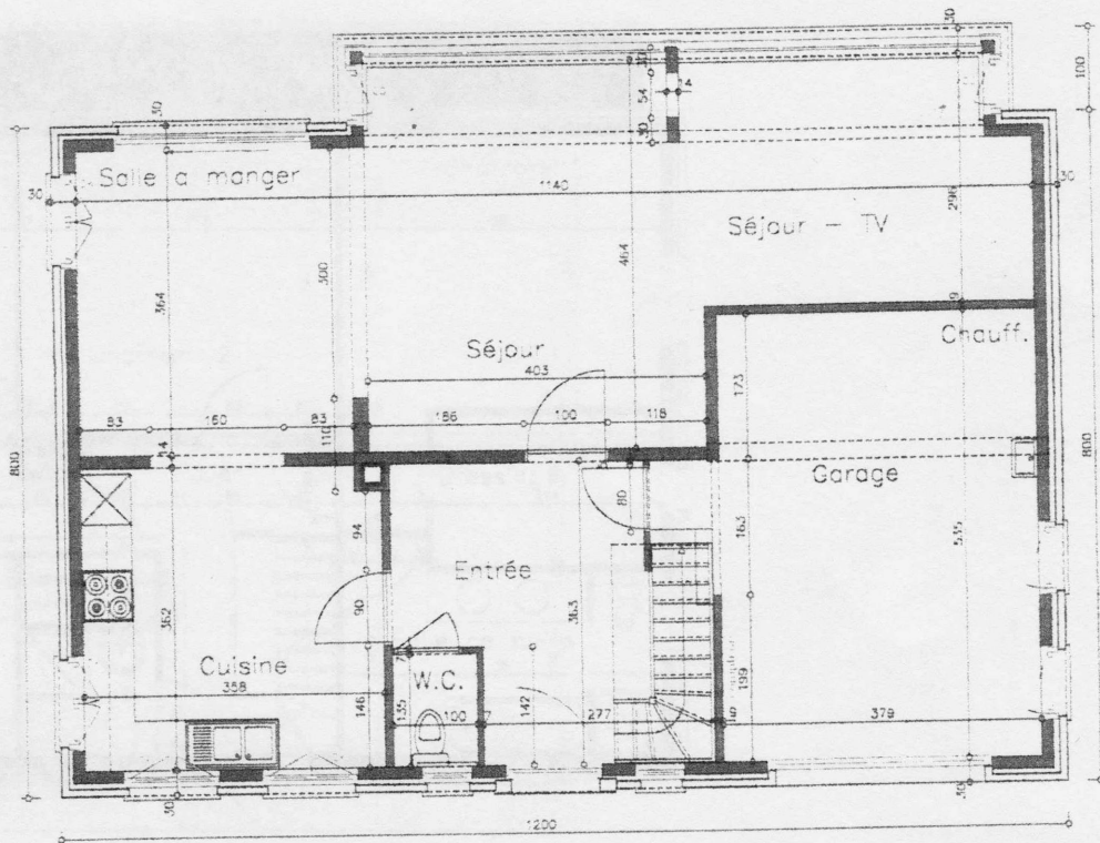
PLAN DE REZ-DE-CHAUSSEE
